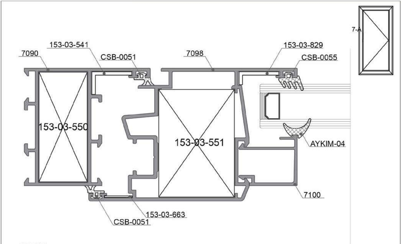
7-A DETAYI DETAIL
