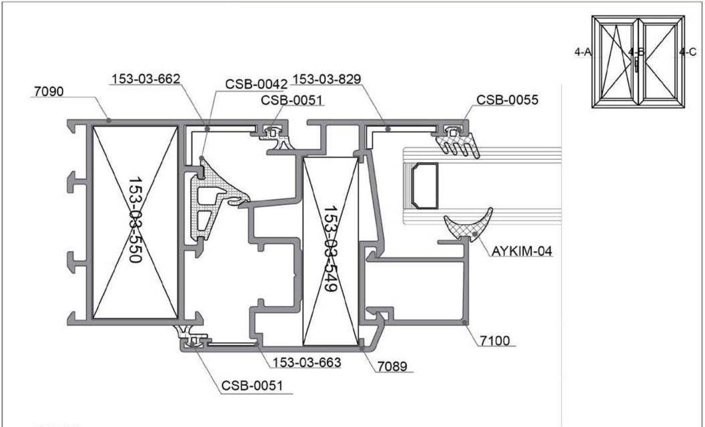
4-A DETAYI DETAIL
