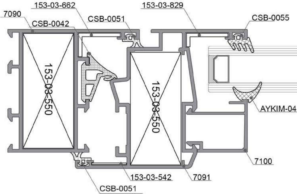
1-A DETAYI DETAIL
