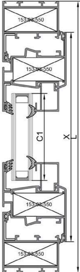
1-A DETAYI DETAIL
