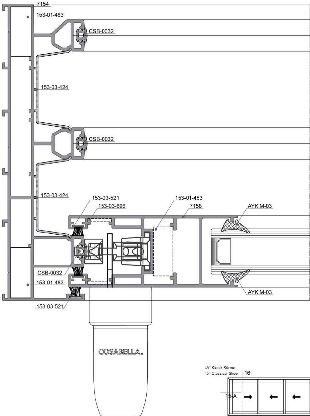
15-A DETAYI DETAIL
