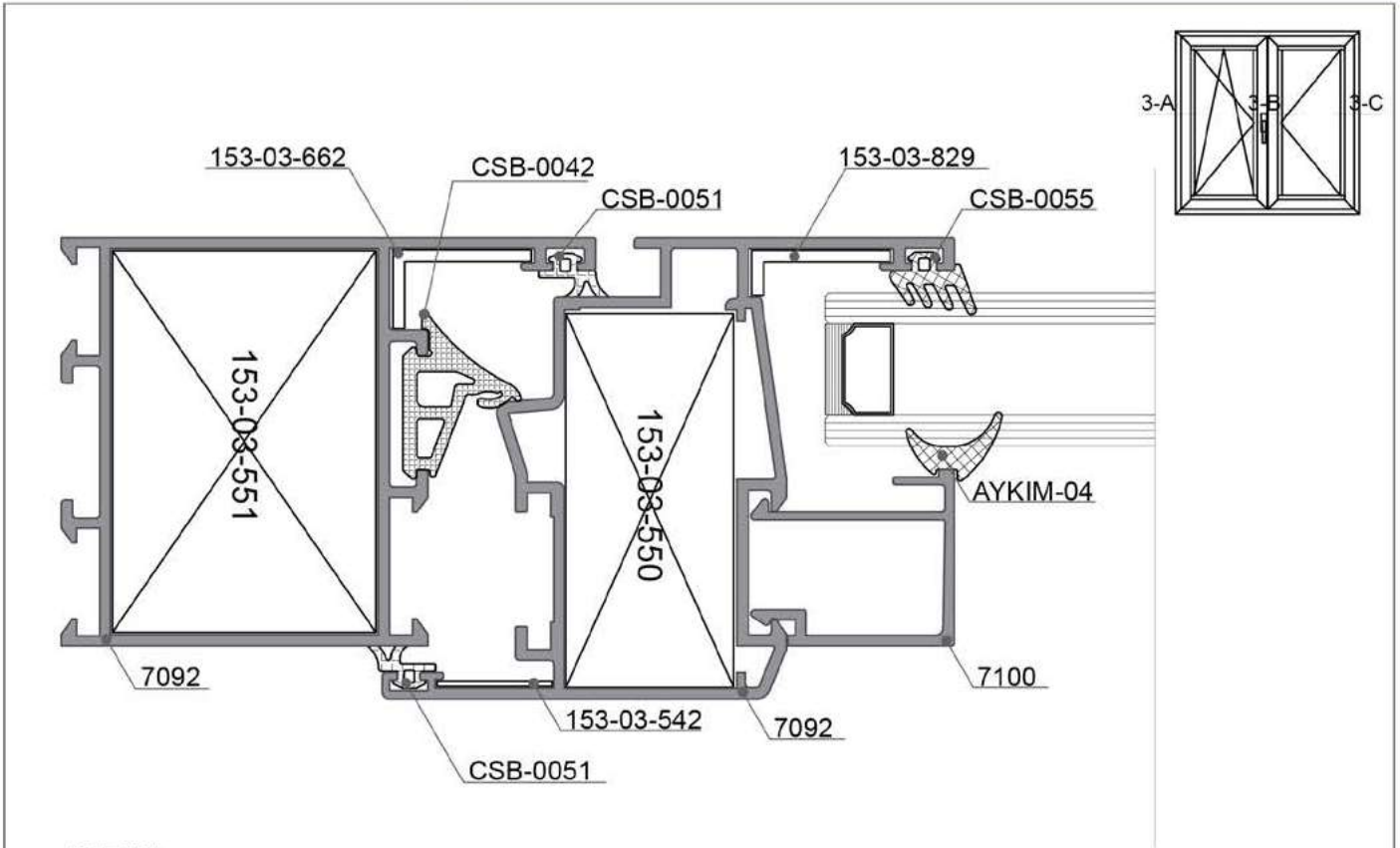
3-A DETAYI DETAIL
